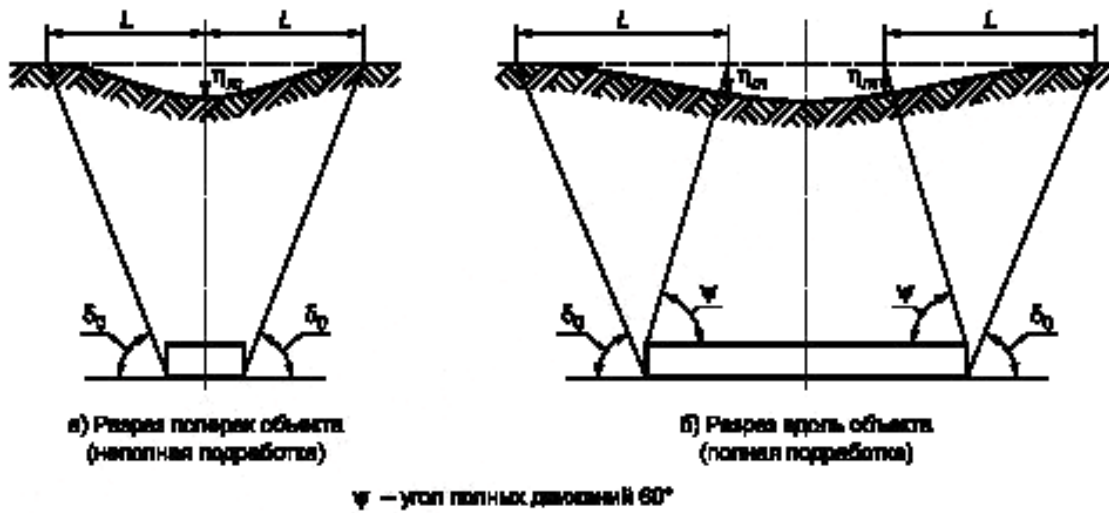
Рисунок Р.1 — Основные параметры мурды сдвижения
