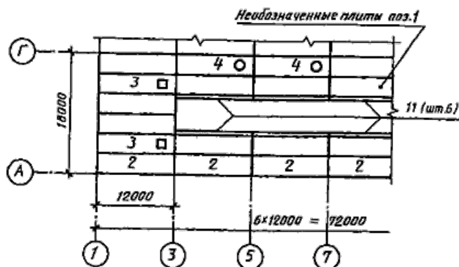
СХЕМА РАСПОЛОЖЕНИЯ ПЛИТ ПОКРЫТИЯ
