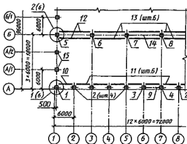
СХЕМА РАСПОЛОЖЕНИЯ КОЛОНН И ПОДКРАНОВЫХ БАЛОК
